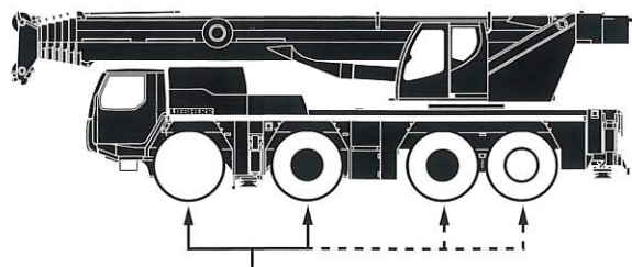
通常操舵軸
